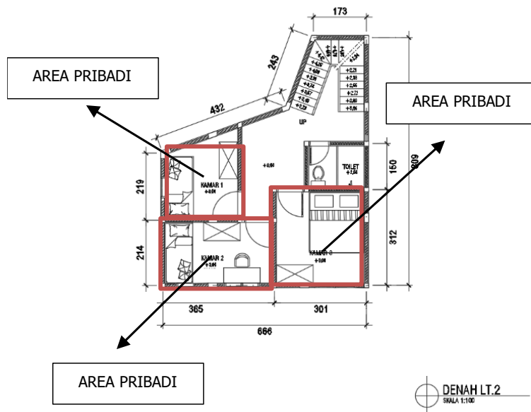
Gambar 3. Denah Lantai 2 dan Mapping Ruang
