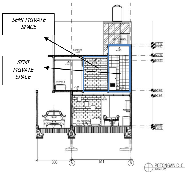
Gambar 4. Potongan C-C dan Mapping Ruang
